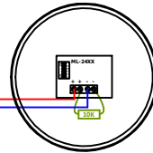
ML - 2420 FLAŞÖRLÜ SİREN KONVANSİYONEL
